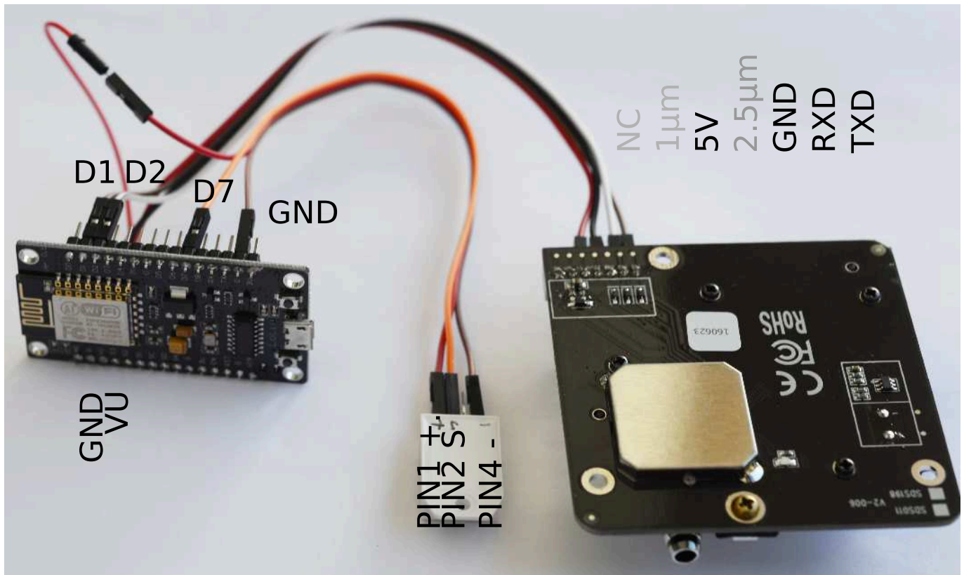
Figure 3: Elektronik zusammgebaut für Station
